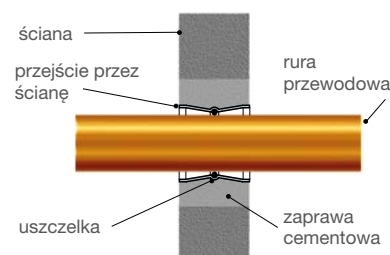
Typowe szczelne przejście przez ścianę
