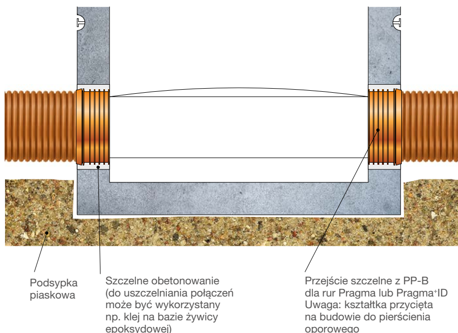
Przekrój przez połączenie studnia betonowego - rura Pragma®
