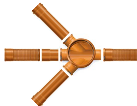
Przykład montażu rur Pragma® z kinetami przelotowymi z PP
