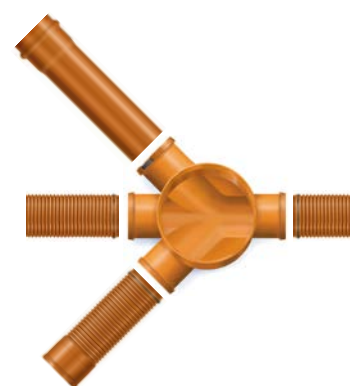
Przykład montażu rur PVC do kinet typu Pragma®.
